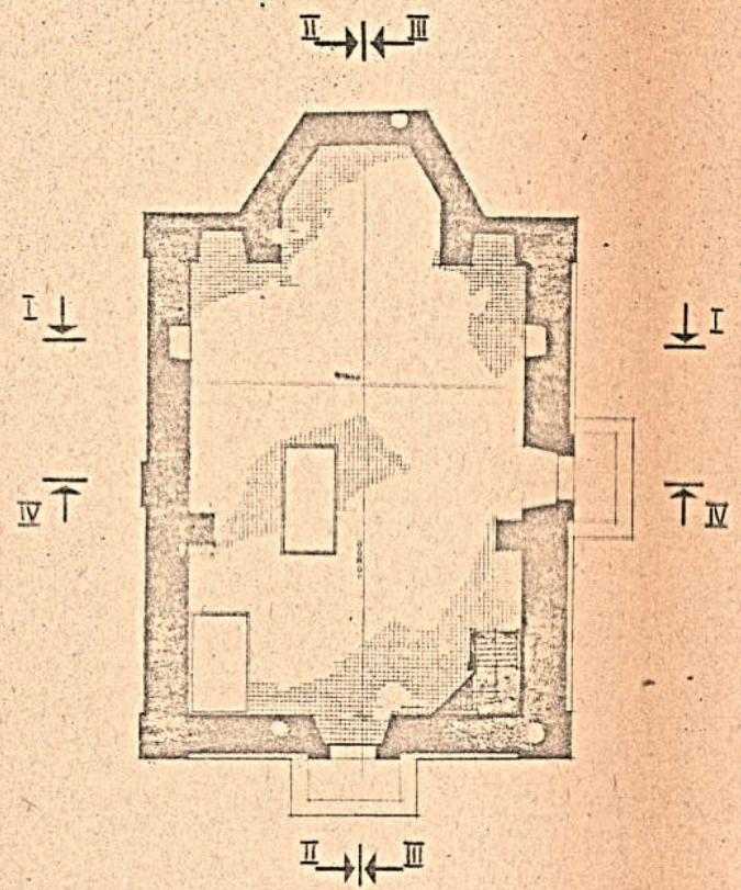
ПЛАН НА ВІДМ. + 1.000 м
