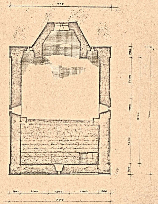
ПЛАН НА ВІДМ. + 3.500 м
