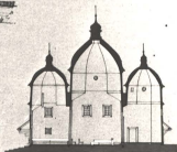
розріз 1-1 М 1:100
